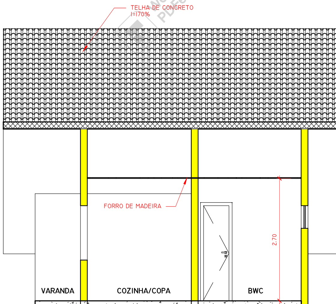
2 CORTE 02 1 : 50
