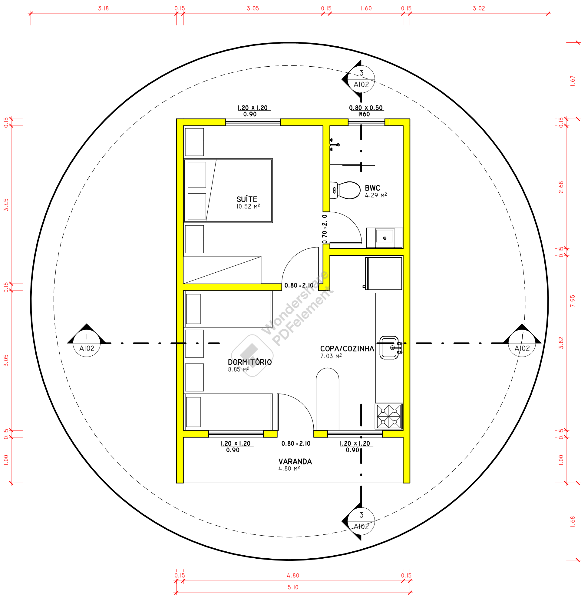
I PLANTA BAIXA - OPÇÃO 03 I : 50
