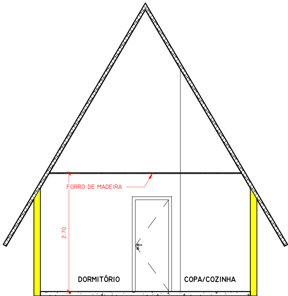
1 CORTE 01 1 : 50
