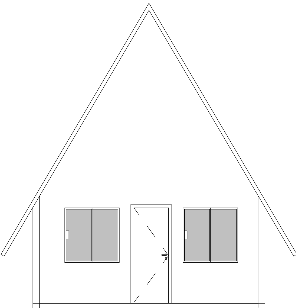
2 FACHADA PRINCIPAL 1 : 50
